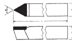
Roscado Estilo E Ángulo Incluido 60°
